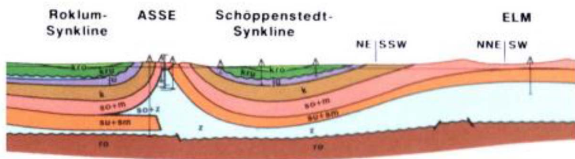
Abb. 5.9: Profil durch den Schmalsattel Asse und den Breitsattel Elm (aus: Geotektonischer Atlas von Nordwestdeutschland, KOCKEL [Hg.] 1996)
